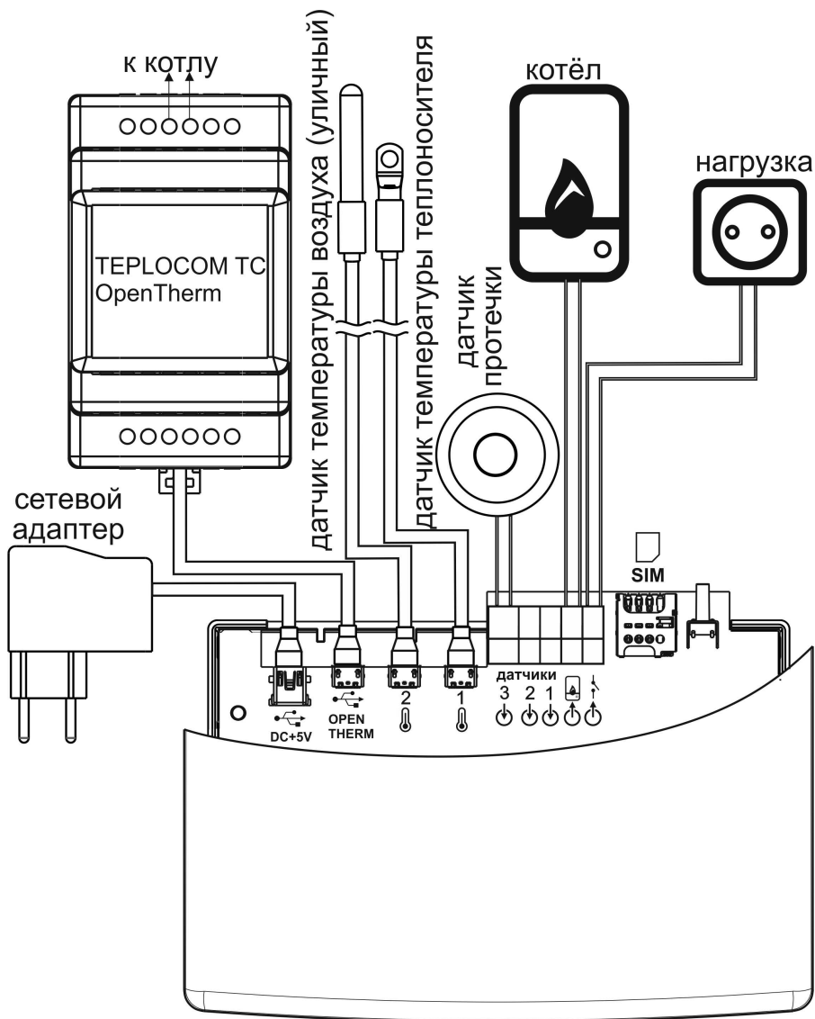
Рисунок 3 - Схема подключений
